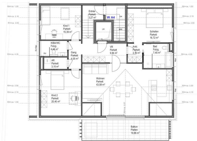
Flächenaufstellung
